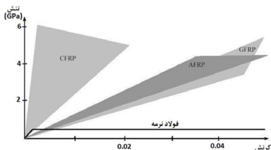
شکل ۱: منحنی‌های تنش-کرنش کامپوزیت‌های FRP در مقایسه با فولاد نرمه [۱]
